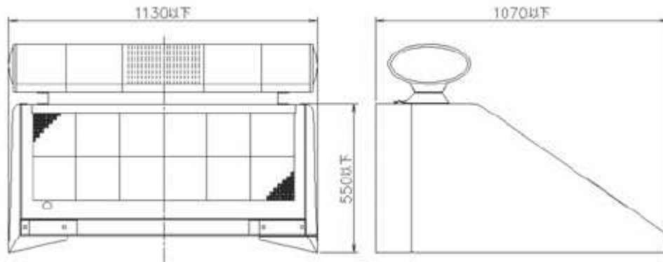
参考図 車載式標識装置 外形図
