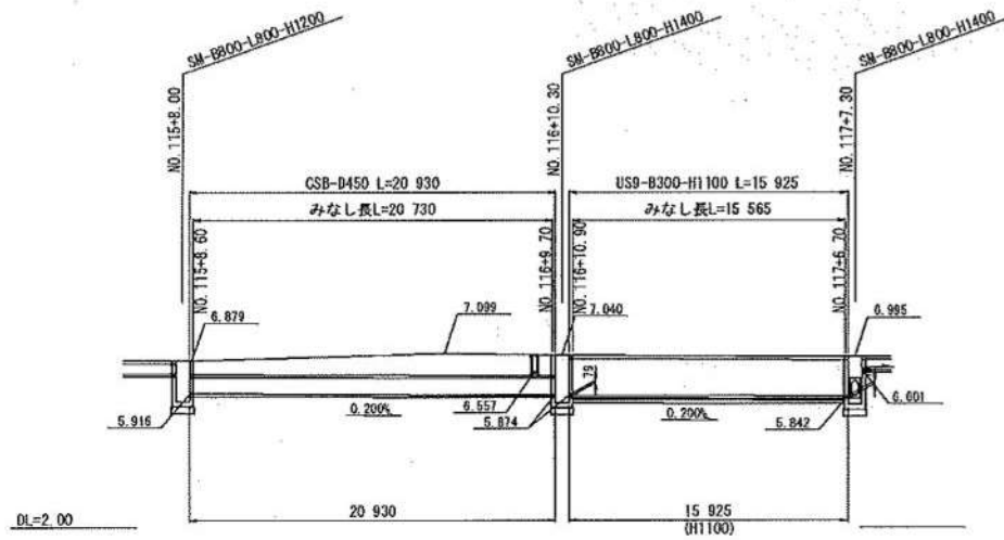
側面図 V=1:10 H=1:200 (NO. 116+10.85~NO. 117+6.75 (R))
