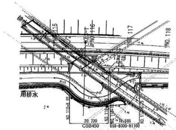
平面図 S=1:500 (NO. 116+10.85~NO. 117+6.75 (R))
