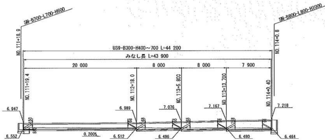
側面図 V=1:10 H=1:200 (NO. 111+19.40~NO. 114+0.40 (L))
