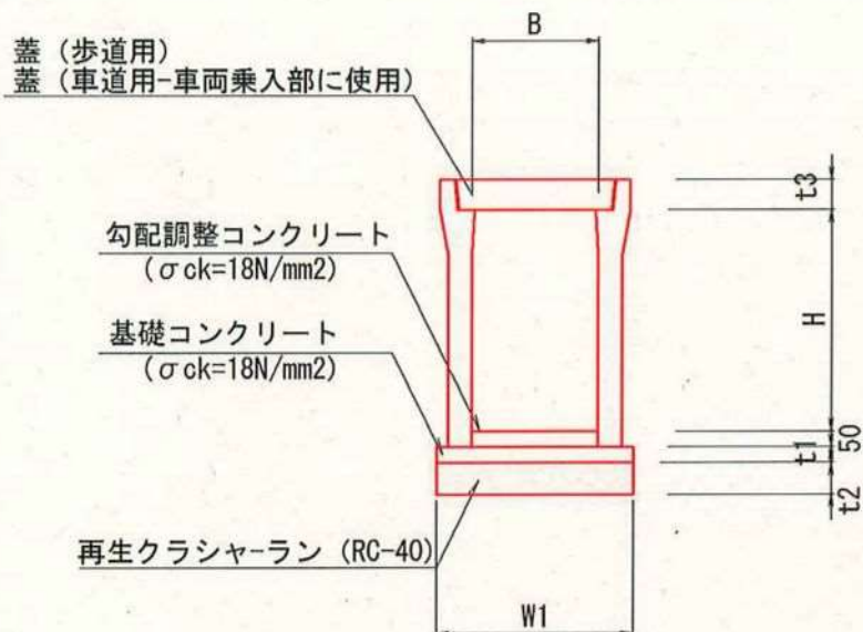
可変側溝一覧表
